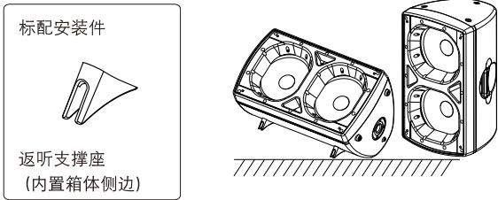
S1200返听安装示意图
