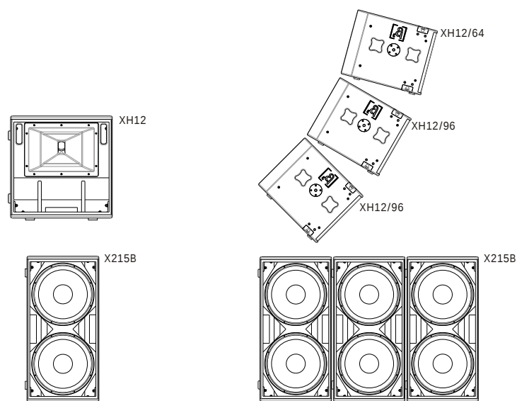
方案2：3只一组吊挂
